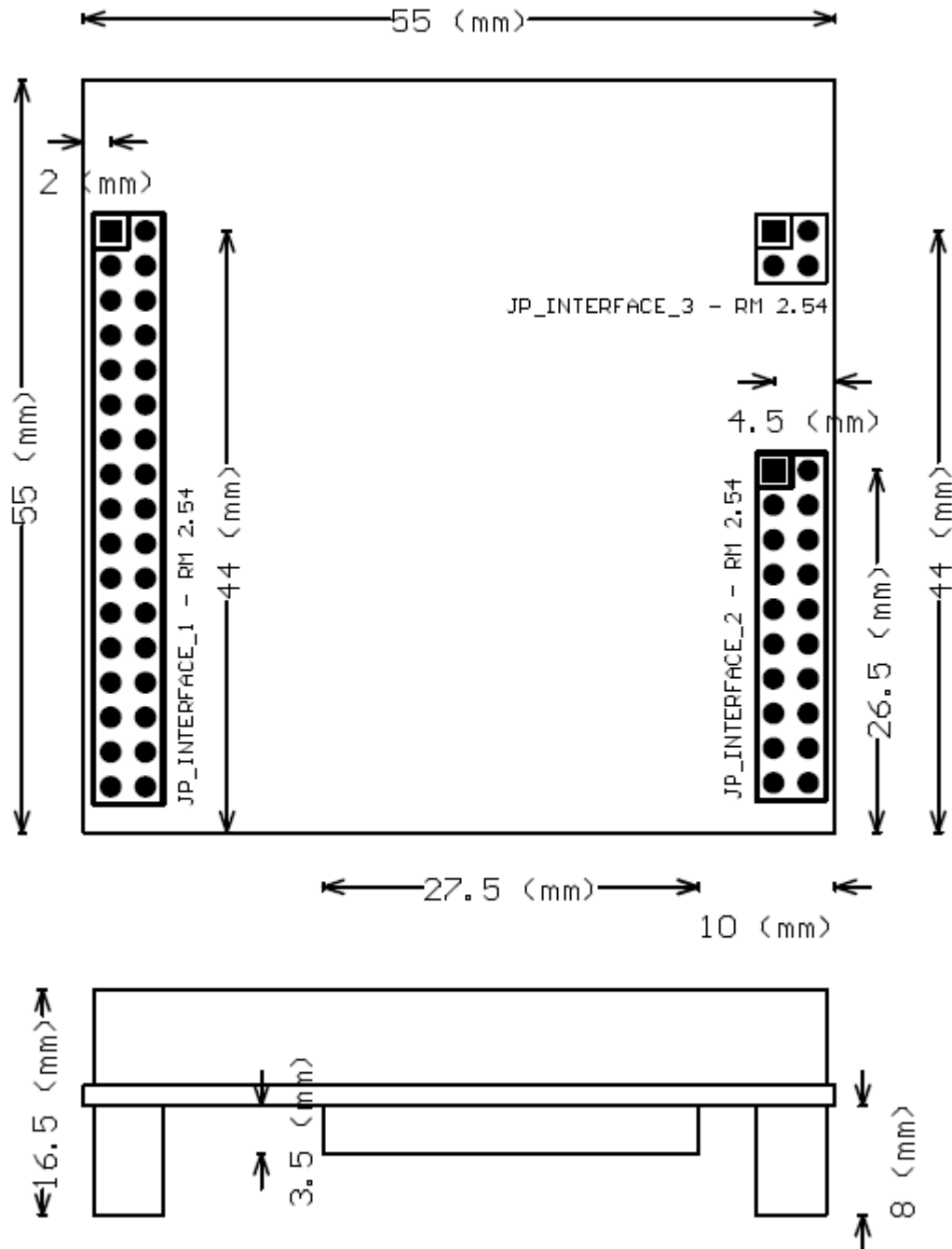
Bild 4.1 Fallguy ULTRA 2 MP3-Modul Rev.C - Abmessungen
