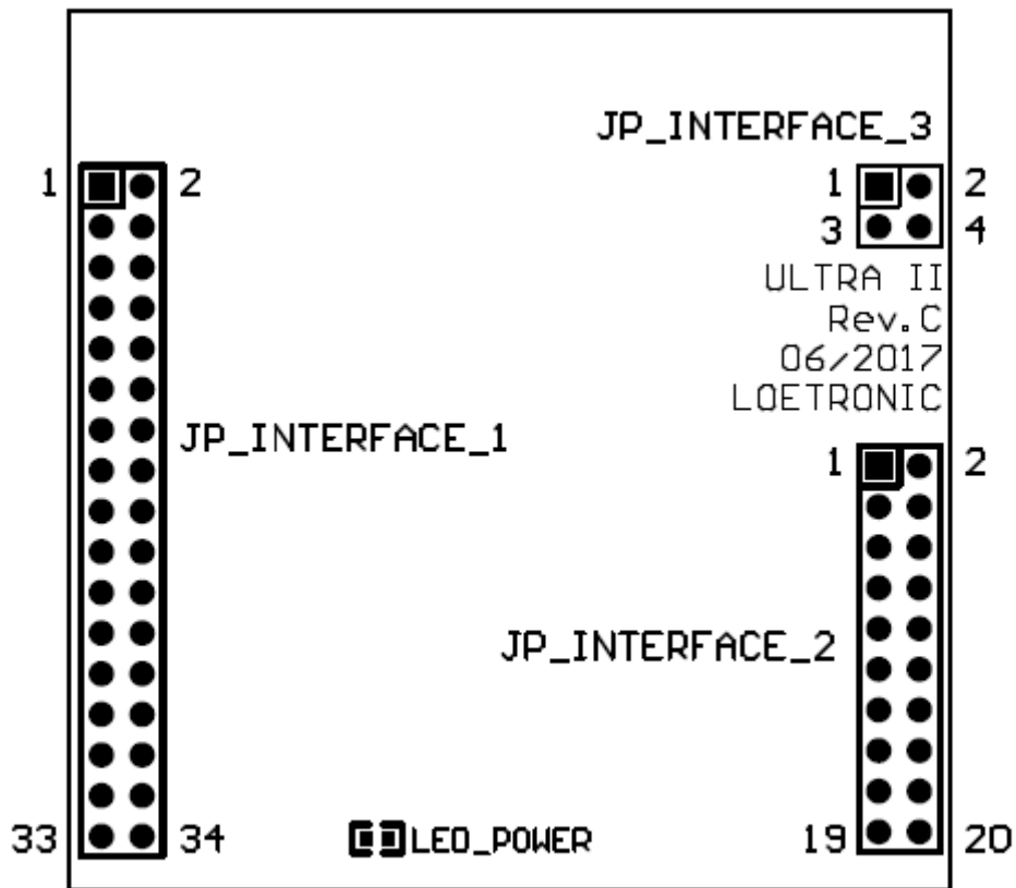
Bild 3.1 Fallguy ULTRA 2 MP3-Modul Rev.C – Anschlüsse
