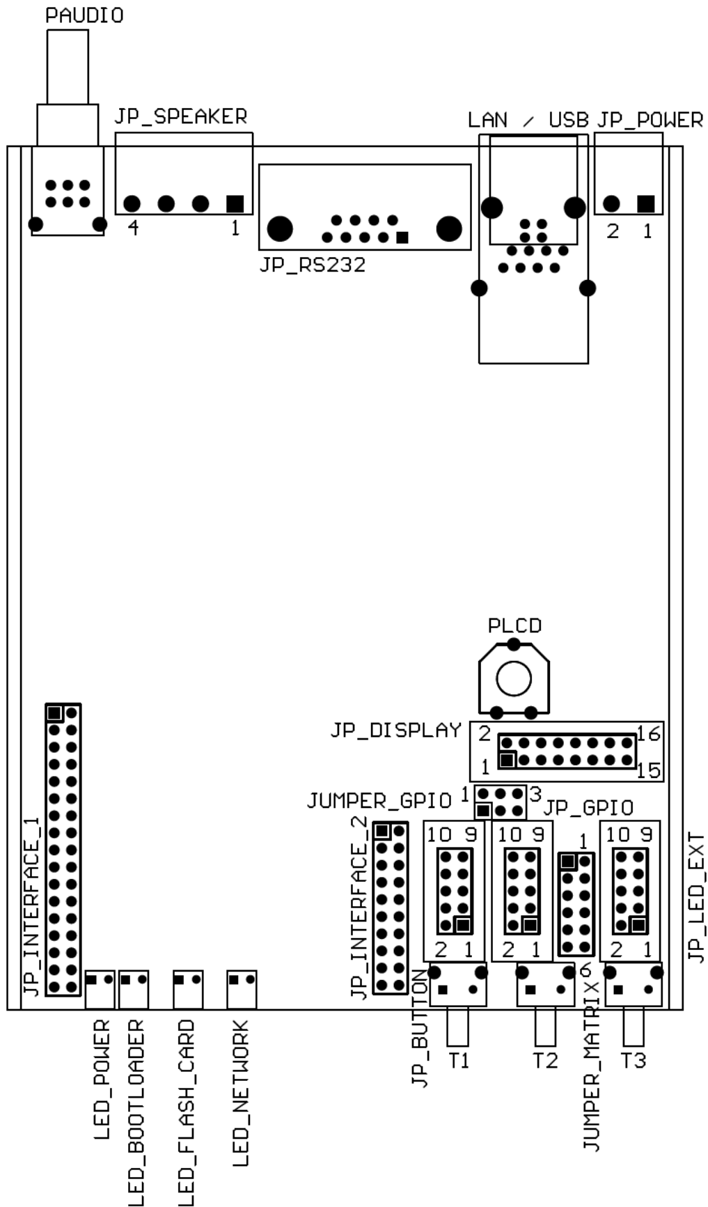
Bild 3.1 Fallguy ULTRA Carrier Board AMPII Rev.F – Anschlüsse und Bedienelemente
