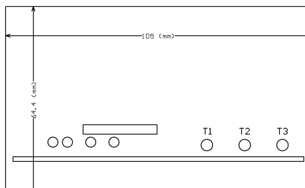
Bild 4.1 Fallguy ULTRA Carrier Board AMP11 Rev.F und ULTRA AMP11 Casing - Abmessungen
