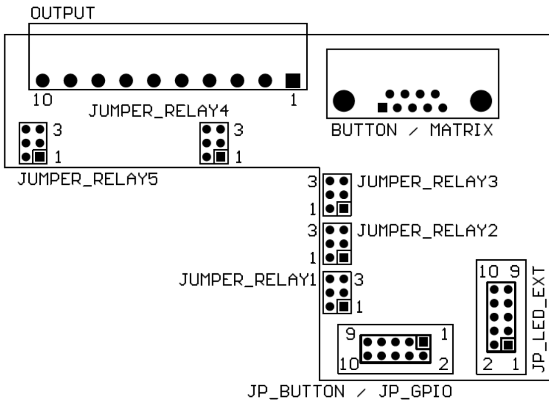
Bild 3.2 Relais-Platine für Fallguy ULTRA Carrier Board AMPII Rev.B – Anschlüsse
