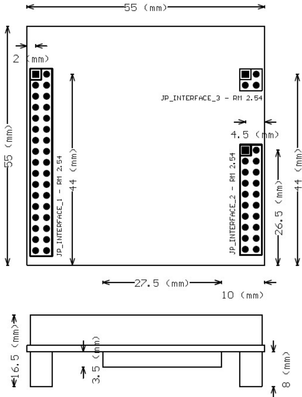
Bild 4.1 Fallguy ULTRA DUAL MP3-Modul Rev.B - Abmessungen
